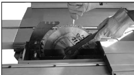
montáž kotouče 305 x 30 x 3 mm (315 x 30 x 3 mm, 254 x 30 x 3 mm)
